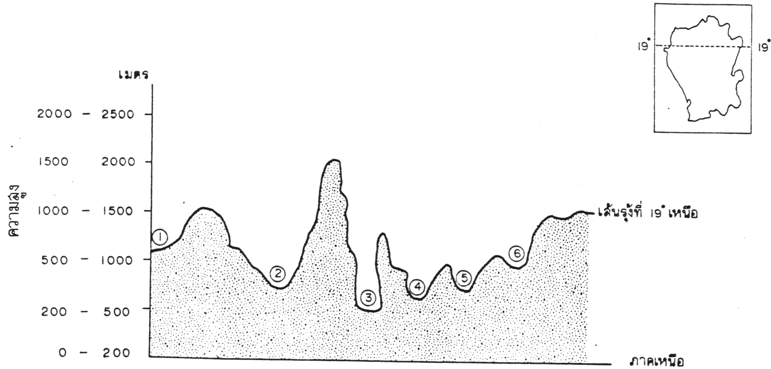
แผนภาพที่ 1 รูปตัดของภาคเหนือตามแนวตะวันตก - ตะวันออก
