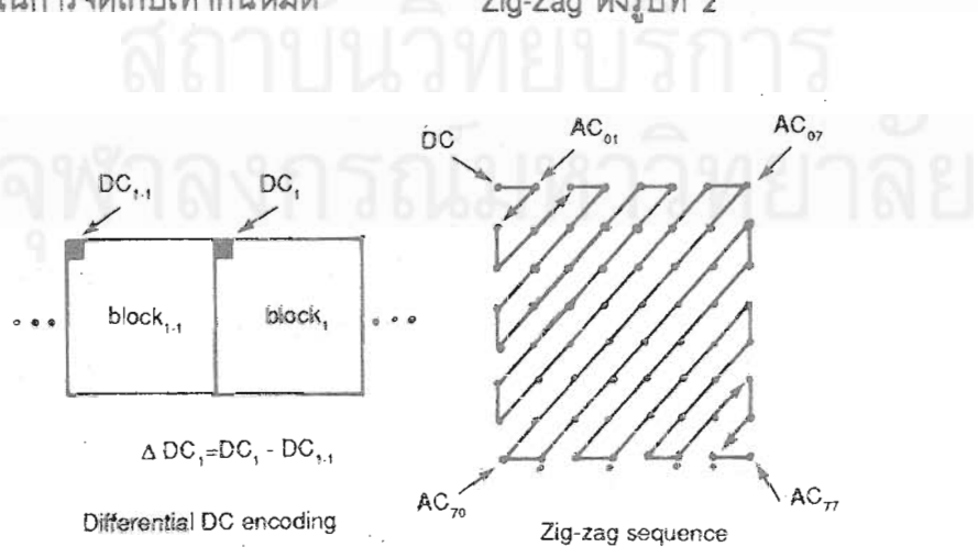
รูปที่ 2 แสดงลำดับการจัดเก็บแบบ Zig-Zag
