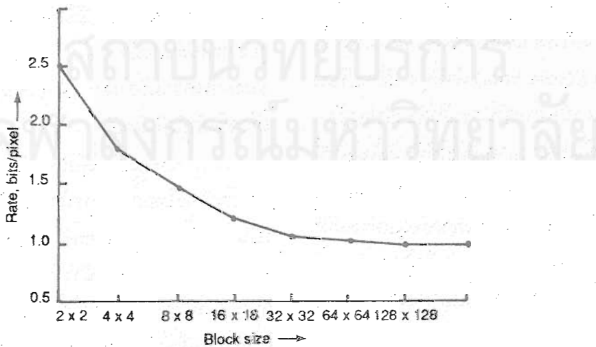
รูปที่ 1 แสดงความสัมพันธ์ระหว่างขนาดของพื้นที่สี่เหลี่ยมย่อยและจำนวนบิตต่อพิกเซลของการเข้ารหัสการแปลงกับข้อมูลที่ได้จากการสุ่มแบบ Gaussian
