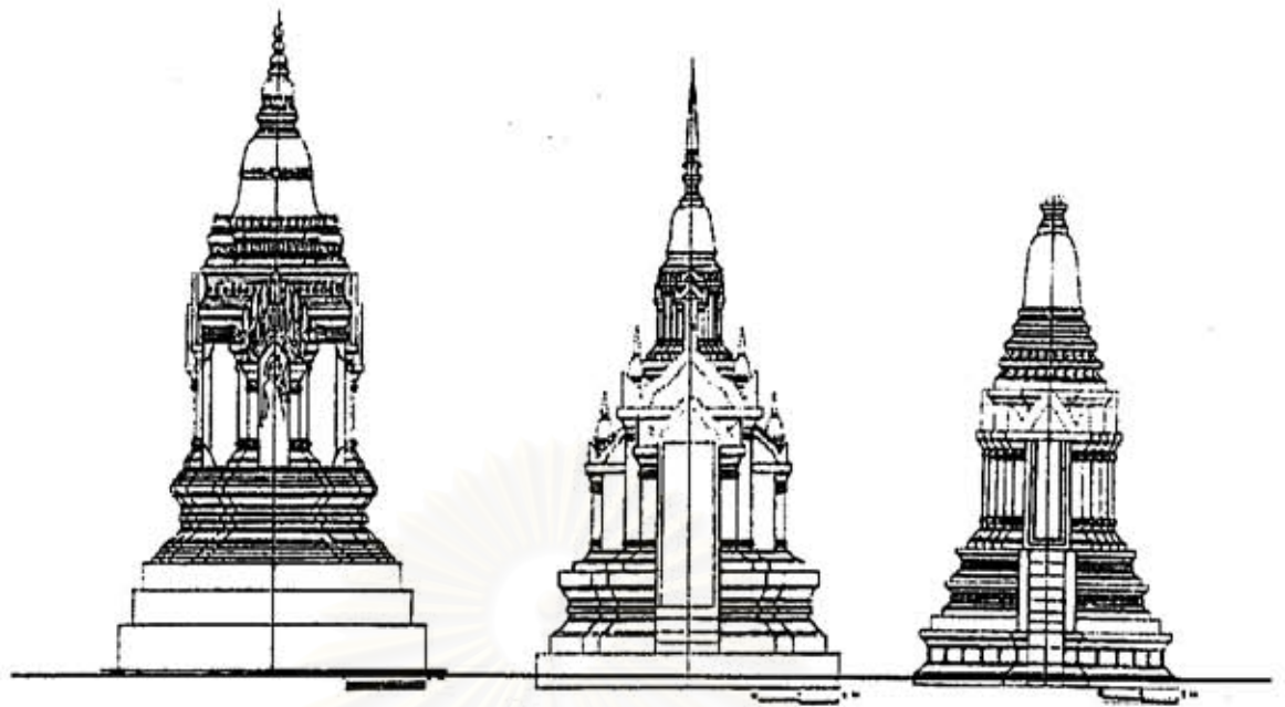
ภาพที่ 7.16 จ. รูปด้านเจดีย์รายวัดเจดีย์เจ็ดแถว
