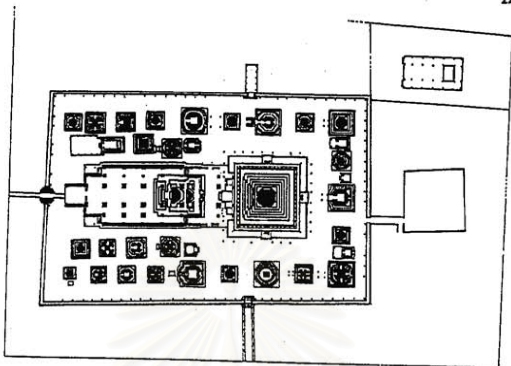
ภาพที่ 7.16 ก. ผังบริเวณวัดเจดีย์เจ็ดแถว
