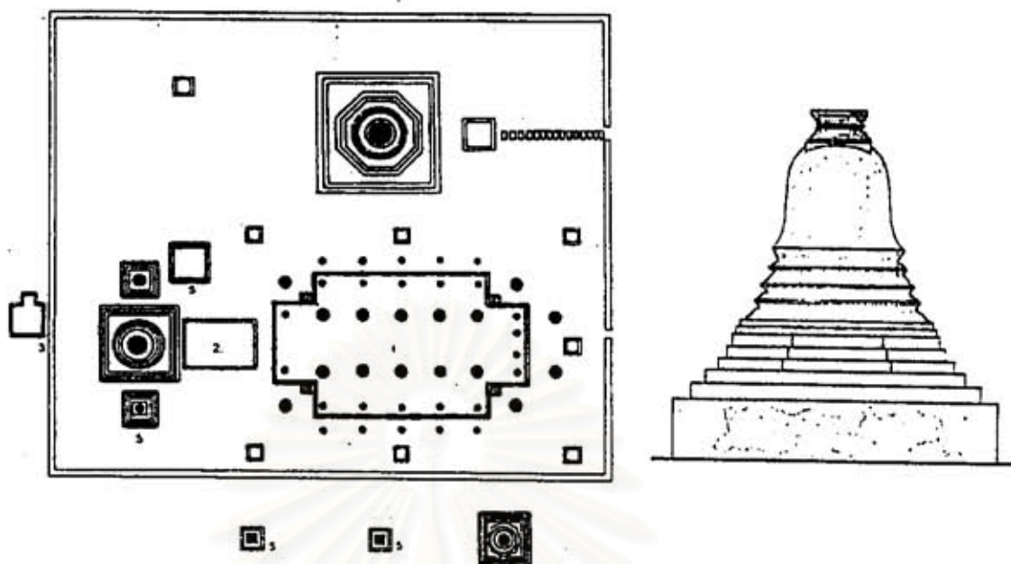
ภาพที่ 7.13 ก. ผังบริเวณวัดมังกกร และรูปด้านเจดีย์ประธานวัดมังกกร
